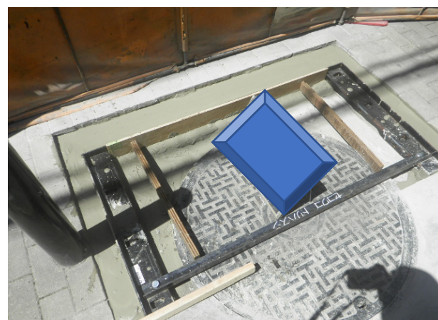
段差解消受枠の設置状況 (コンクリート打設後)
